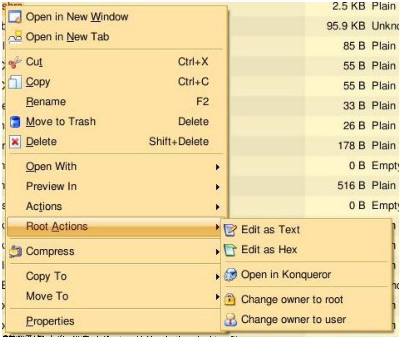
RootActions 2.4.3-1mib2009.1.i686
